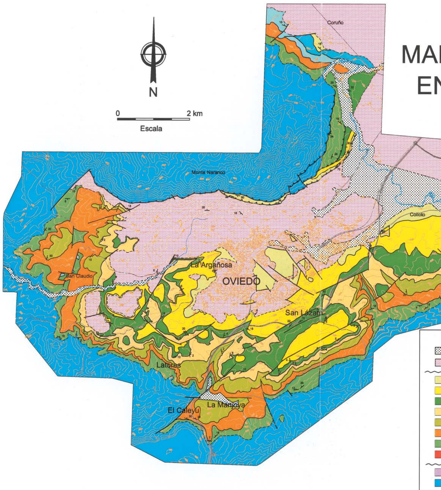
Figura 3. Mapa geológico del Cretácico del sector occidental de la “Depresión mesoterciaria central” (zona comprendida entre Oviedo y Pola de Siero).
