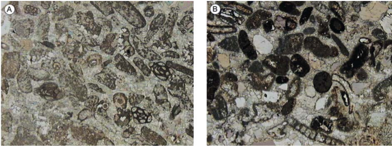
Figura 22. Microfacies características de la Formación Oviedo (longitud de la barra igual a 1 mm). A) Caliza grainstone bioclástica. Entre los bioclastos son frecuentes las algas ( Halimeda , Acicularia ), foraminíferos (miliólidos), lamelibranquios, gasterópodos y crinoideos. B) Caliza grainstone con algas ( Halimeda ), foraminíferos y algo de cuarzo.
