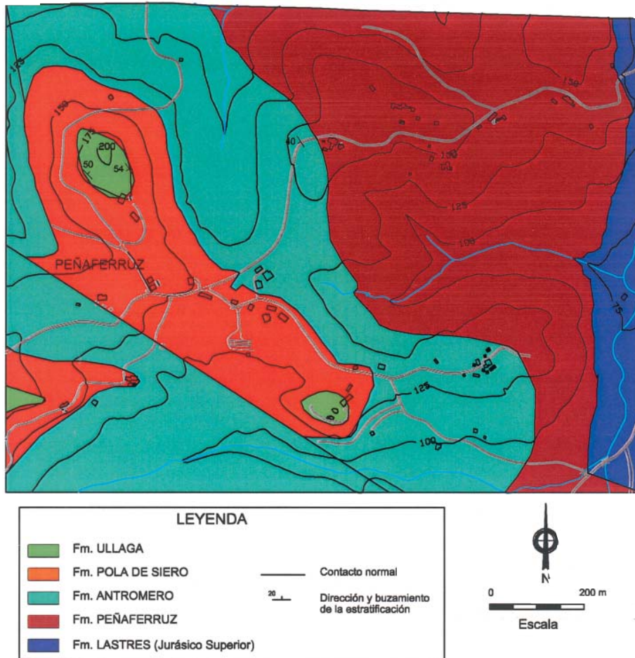
Figura 4. Mapa geológico del sector de la "Franja móvil intermedia" correspondiente al entorno de Peñaferroz (Gijón).
