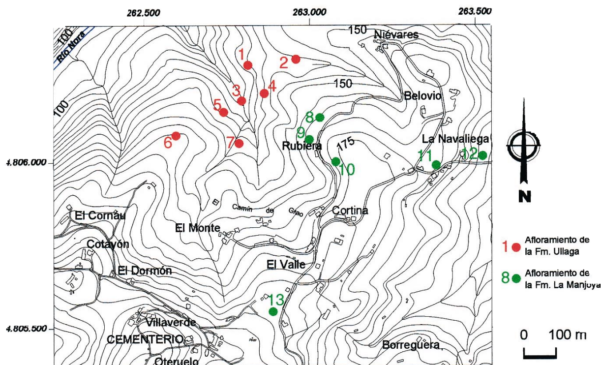
Figura 9. Afloramientos de las formaciones Ullaga y La Manjoya en el oeste de San Claudio.
