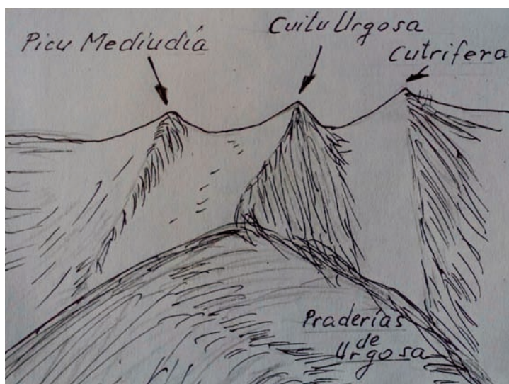
Gráfica explicativa de la fotografía anterior (según dibujo del autor)
