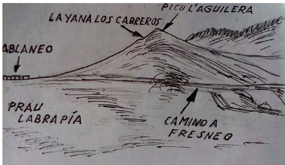
Gráfico ilustrativo de la foto anterior, que representa el entorno de Ablaneo (según dibujo del autor).
