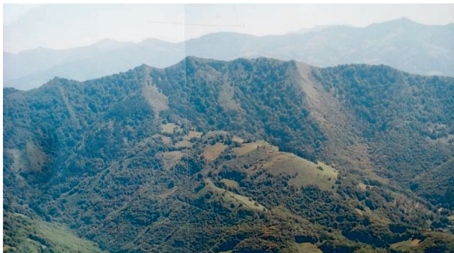
Cordal de Llongalendo. La orientación geográfica de la fotografía es la siguiente: el sur está al fondo y el Picu Mediudía es la cumbre situada a la izquierda. Para dar una idea al lector, diremos que si nos desplazamos en la imagen, a través del cordal, de derecha a izquierda, estaremos haciendo el recorrido de oeste a este.
